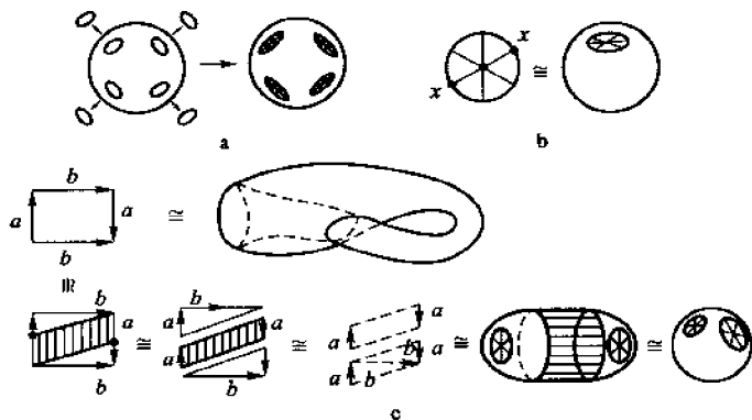
图 5 a) 流形 M_\mu^2 = S^2 + (\mu) (图中 \mu = 4 ), 由球面 S^2 附加 \mu 个默比乌斯带得到;
