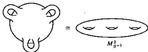
图 4 具有 g 个环柄的球面 S^2 + (g) = M_g^2 (图中 g = 3 )
