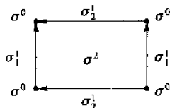
图 23 环面
