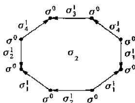
图 26 双环面
