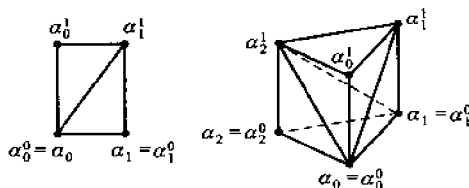
图 35 剖分柱形为单形
