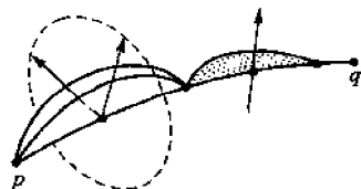
图 111 指数 \lambda=3 . 这个测地线 \gamma_0 对应于三维胞腔 \sigma^3
