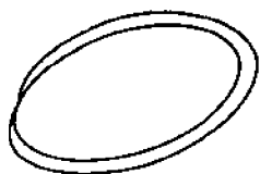
图 113 二重测地线
