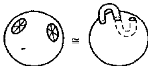
图 7 具有内外翻转环柄的球面 S^2
