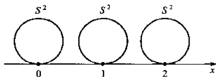
图 45 作用为 x \mapsto x+1
