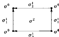
图 24 克莱因瓶 K^2
