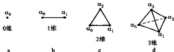
图 2 单形
