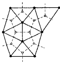
图 42 M^2 的原来的剖分以实线表示; 对偶的剖分则以虚线表示
