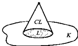
图 37 K \cup CL
